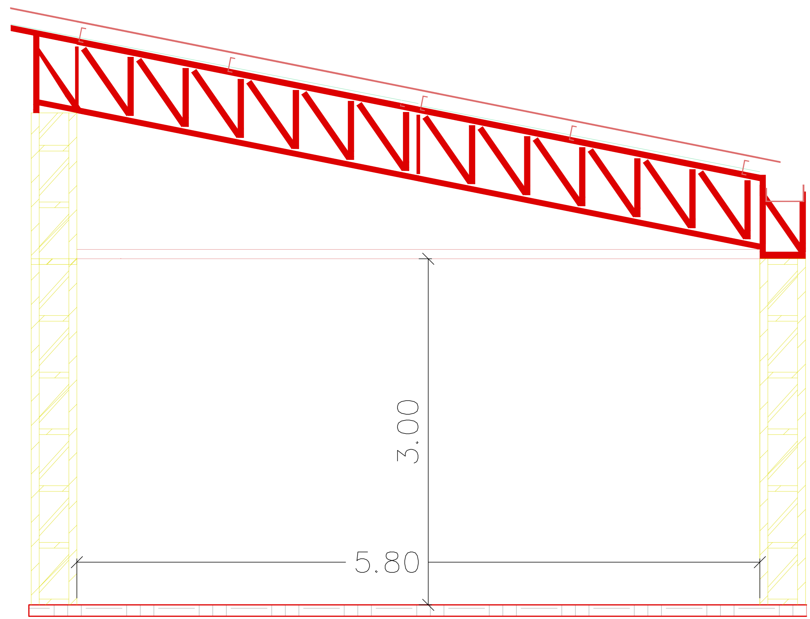
CORTE TIPO AA 1:20
